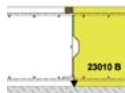
Selbststehend mit Verzahnungsfuge nach DIN-Norm
