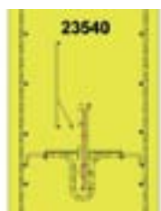
Sollrissfuge flach, mit Fugenblech oder Fugenbandführung
